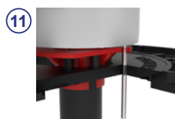
Arretierungsstift für Hülrohrkappe bzw. DALMINEX-Tragplatte Material: 1.4301
