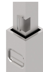
④ Auszugssicherung Transport lock
